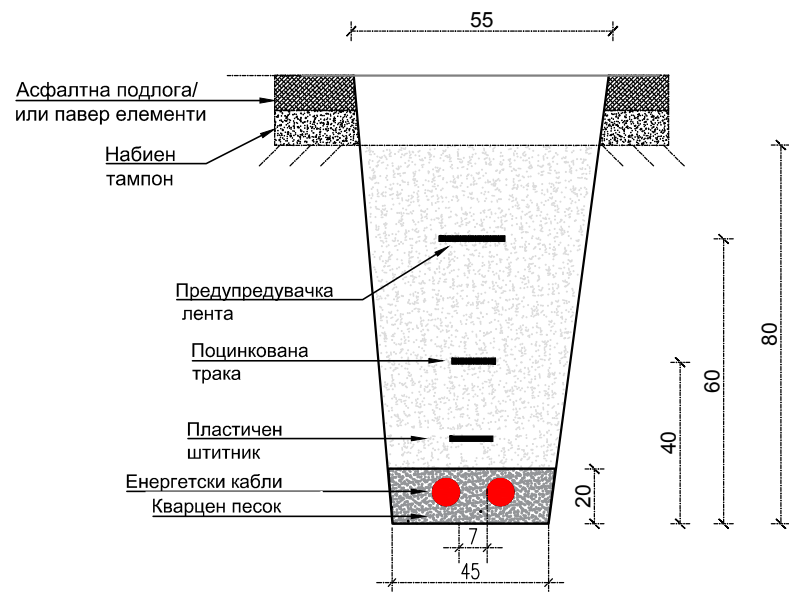
Елементи на кабелски ров
