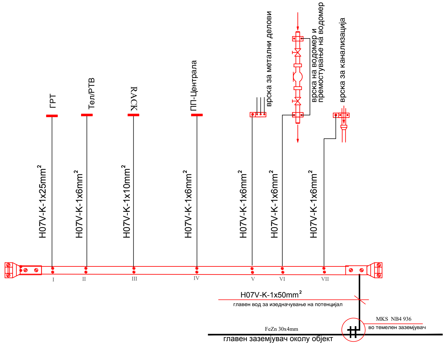
Дополнително изедначување на потенцијал
