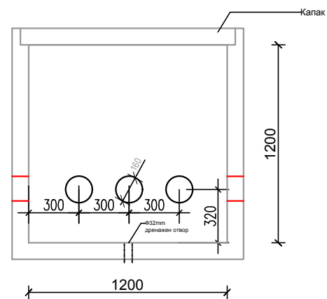
Кабелска шахта-пресек 1:1
