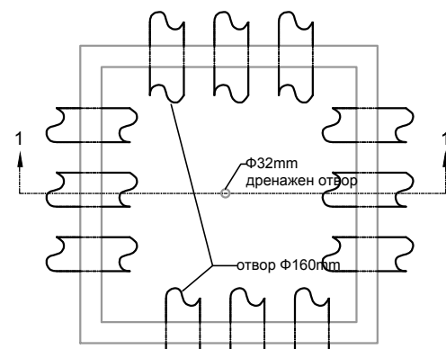
Кабелска шахта-поглед од горе
